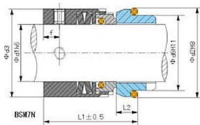
Торцевые уплотнения BS-M7N - аналог уплотнения Burgmann M7N
